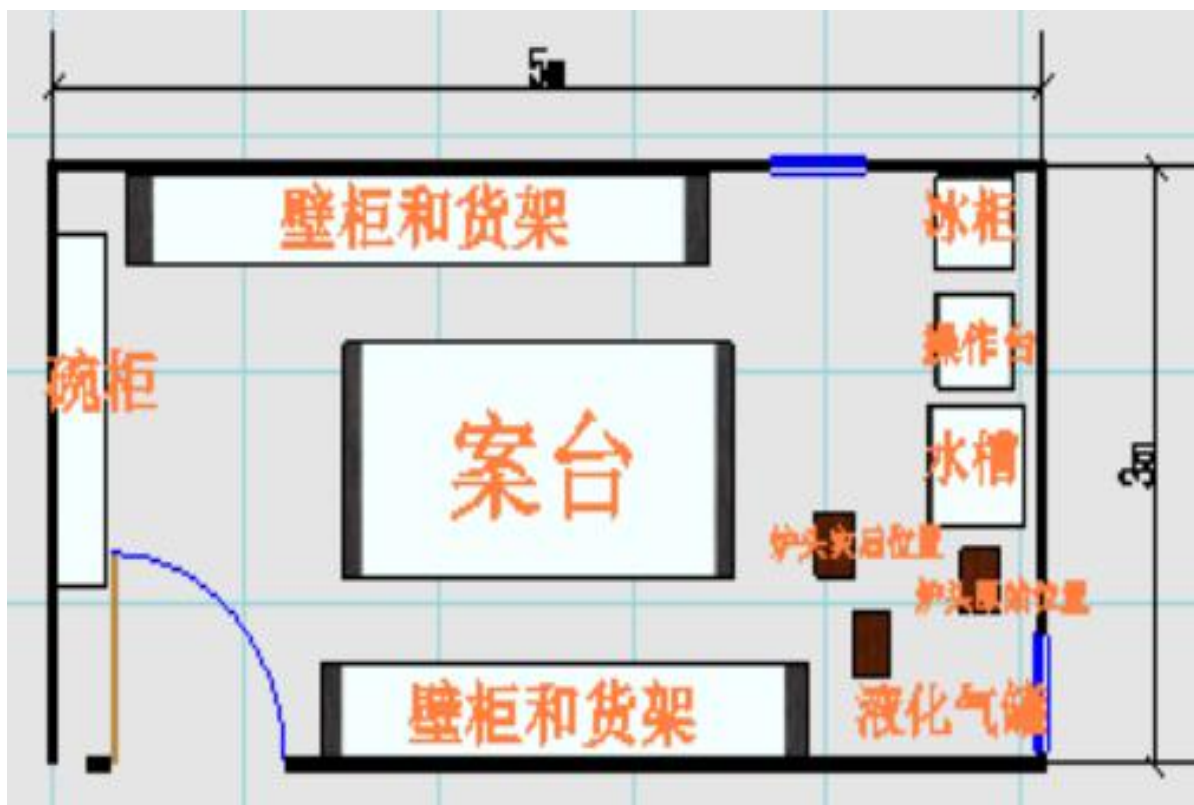
图 3.1.1：厨房平面示意图
